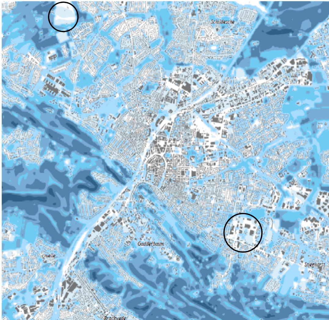
Karte der Kaltluftproduktion, Zukunft (Ausschnitt)
